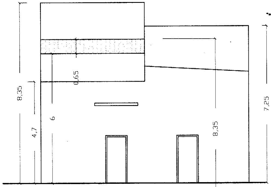
PROSPETTO OVEST b c
