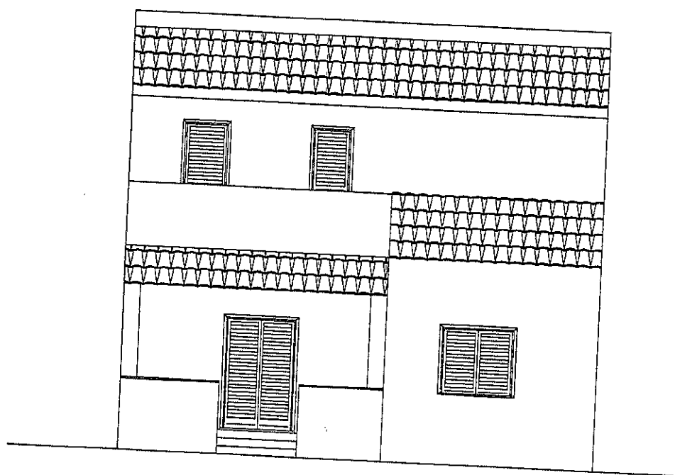
PROSPETTO PRINCIPALE
