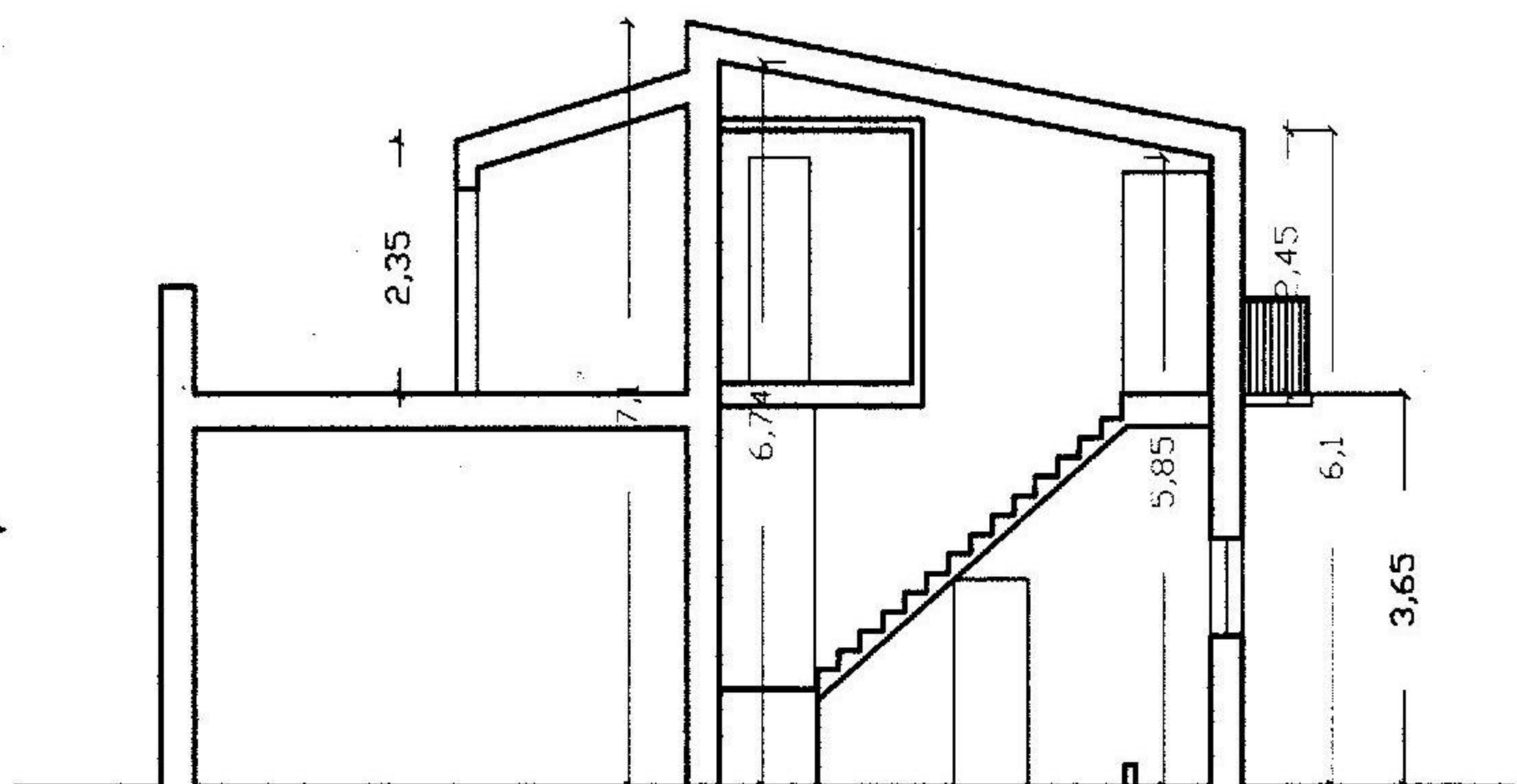
SEZIONE B1-B1
