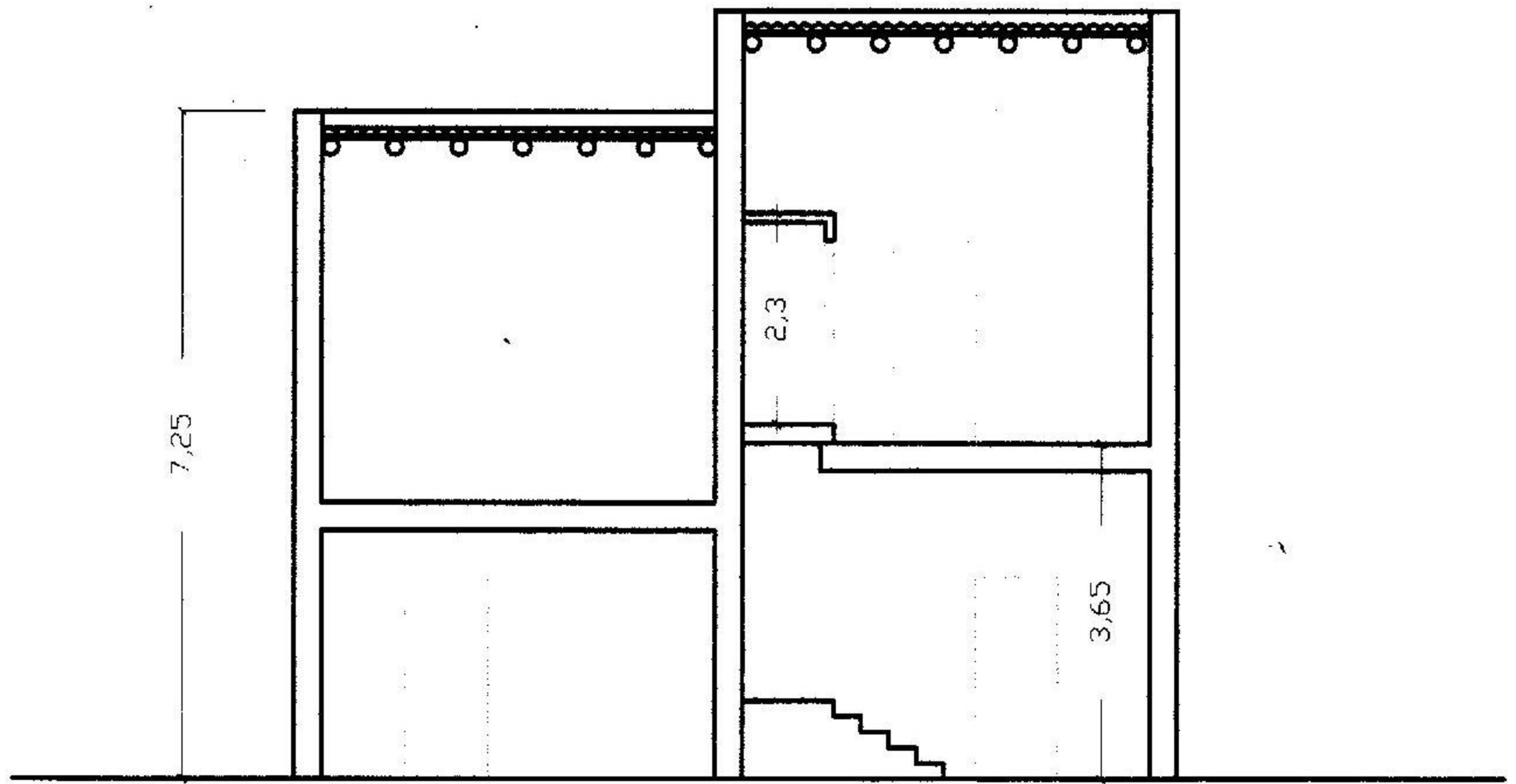
SEZIONE A+A
